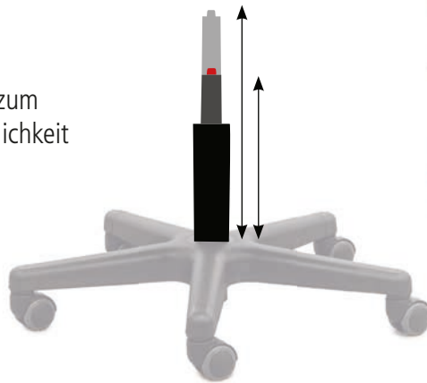
Teleskopgasfeder 12 cm Verstellbereich
