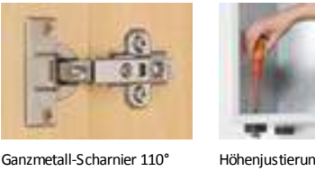
Ganzmetall-Scharnier 110° Höhenjustierung
