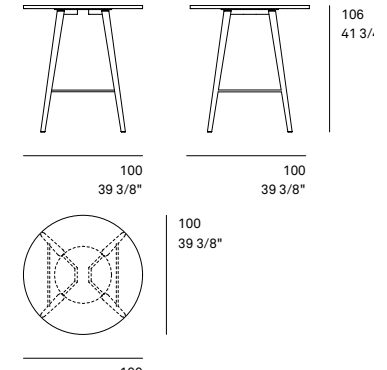
222/71 Rund
