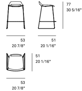
223/10 Barstuhl
