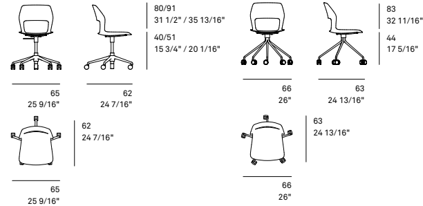
221/00, 221/01, 221/02 Drehstuhl, höhenverstellbar
