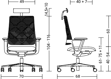
cnx89 / cnx88 mit Armlehne with arm supports 20 kg / 18 kg
