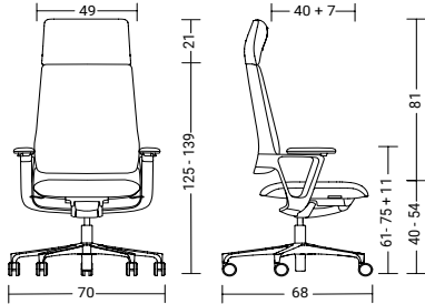
cnx95 mit Armlehne with arm supports 22 kg
