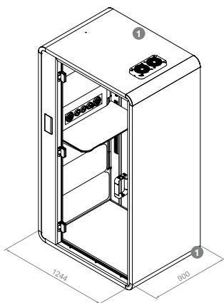
1 Kabelzuführung
