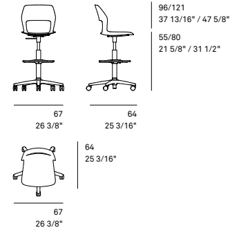
221/50, 221/51, 221/52 Counterstuhl, höhenverstellbar
