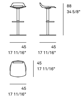
223/90, 223/91 Barstuhl, höhenverstellbar
