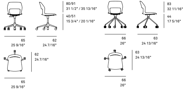
221/00, 221/01, 221/02 Drehstuhl, höhenverstellbar
