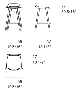
223/20, 223/21 Barstuhl
