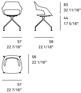
222/30, 222/31, 222/32 Besucherstuhl
